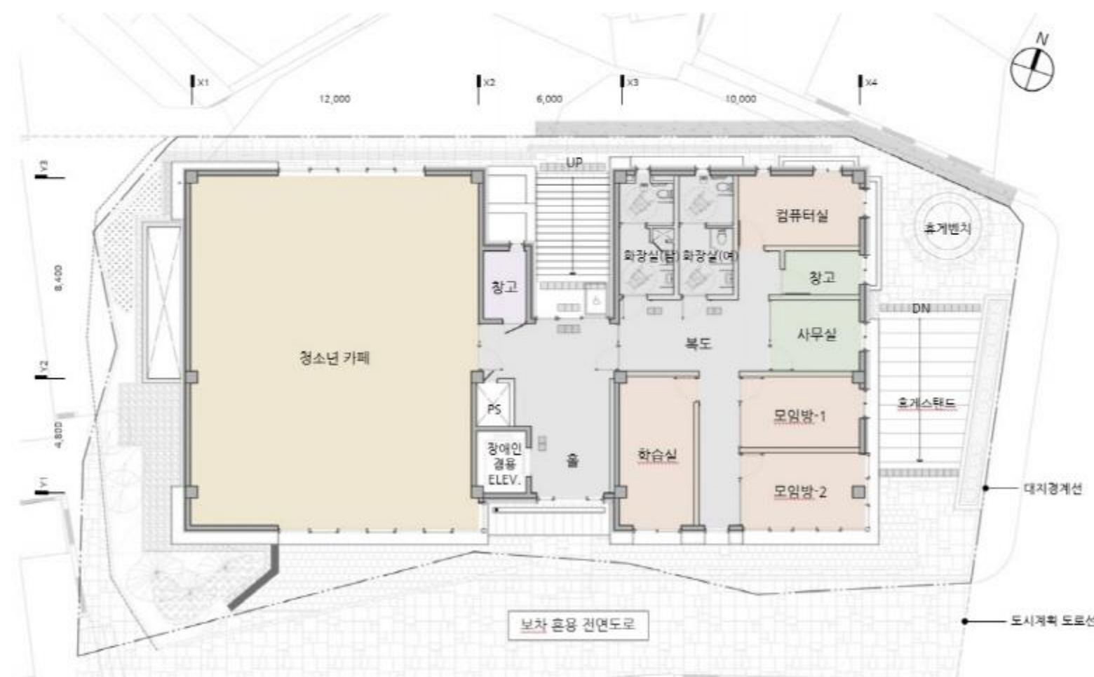
2층 평면도
