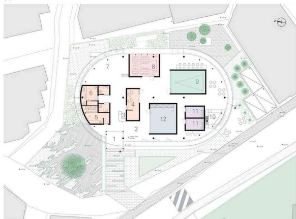
평면도
