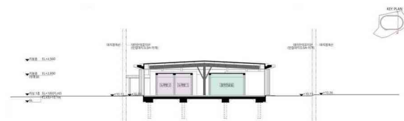
단면도 1
